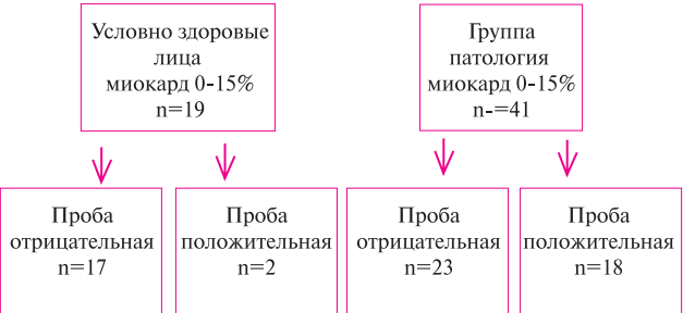
Рис. 4 Результаты пробы с приседанием у лиц с нормальными значениями “миокард”.
