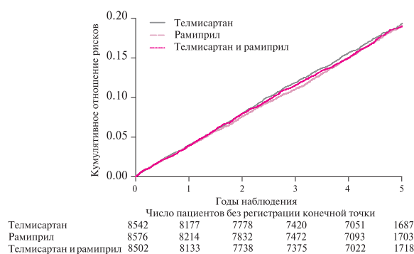
Рис. 3 В исследовании ONTARGET кривые Каплана-Мейера для основной конечной точки (сердечно-сосудистая смерть, ИМ, МИ либо госпитализация в связи с СН) достоверно не различались при лечении телмисартаном (Микардисом), рамиприлом (Altace) и комбинацией этих препаратов [61].
