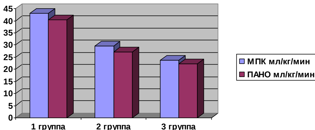
Рис. 2. Сравнительная характеристика спектральной мощности ЭЭГ и данных эргоспирометрических показателей.
