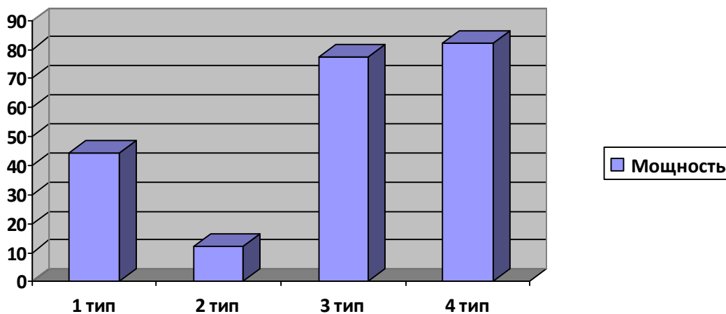
Рис. 1. Значения суммарной мощности спектров в четырех типах картограмм
