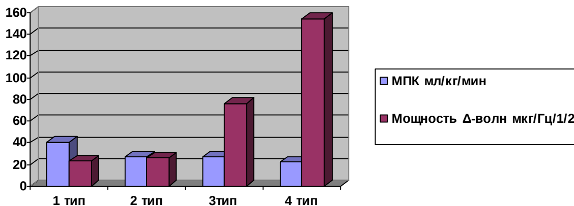
Рис. 3. Характеристика взаимосвязи показателей МПК и спектральной мощности медленноволновой активности мозга
