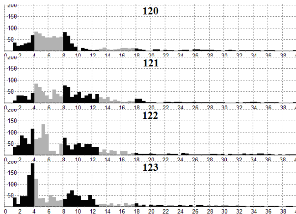
Рис. 3. Спектральная мощность \delta -, \theta -, \alpha -, \beta - и \gamma -ритмов в односекундных отрезках ЭКГ на 120-123 секундах фибрилляции желудочков. \delta -, \alpha - и \gamma -ритмы выделены черным цветом на спектрограммах; \theta - и \beta -ритмы выделены оттенком серого. По оси абсцисс – частота, Гц; по оси ординат – мощность, мкВ
