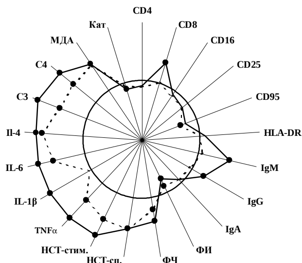
Рис. 2. Показатели иммунного, цитокинового и антиоксидантного статусов у больных ХСО до и после традиционного лечения + деринат + токоферол. Обозначения: 1 – радиус окружности – показатели здоровых доноров (1 группа); 2 – ———— – показатели больных ХСО после традиционного лечения + деринат + токоферол (2 группа); 3 – — · — · — · — – показатели больных ХСО после традиционного лечения + ридостин + эспа-липон (3 группа); 4 – ● – p < 0,05 между показателями 2-3 групп по отношению к 1 группе.
