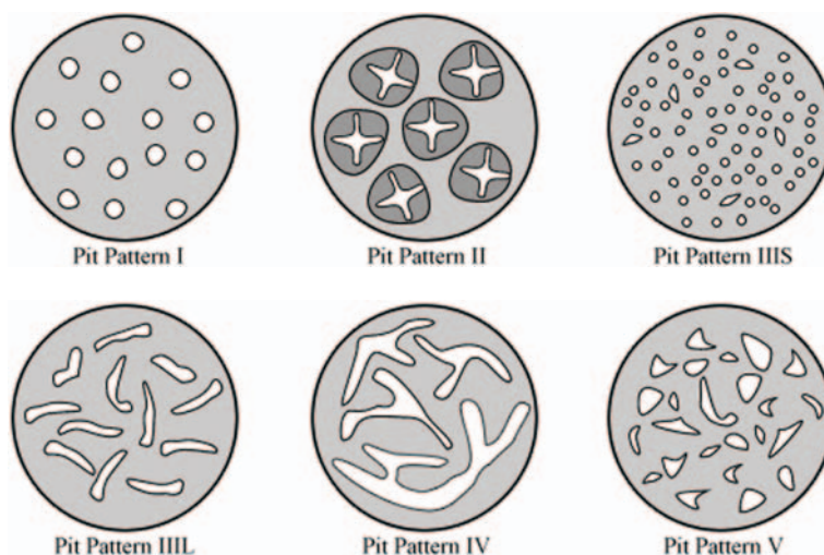
Рис. 1. Классификация структуры микрорельефа Pit Pattern [6]: I. Круглые (нормальные) ямки; II. Звездчатые ямки; III с . Трубчатые или круглые ямки меньше, чем нормальные ямки (тип I); III л . Трубчатые или круглые ямки больше, чем нормальные ямки (тип I); IV. Дендритные или извилистые ямки; V. «Разрушенный» рельеф
