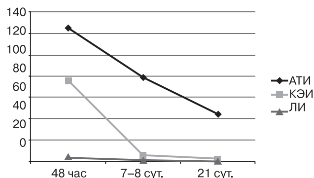
рис. 5: Изменение объема поражения по данным МРТ-перфузии (МТТ-карта, в см³)
