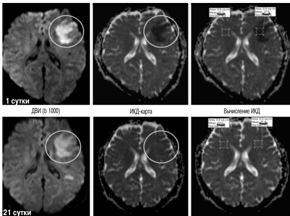
рис. 1: ДВ-МРТ у больного с ИИ в динамике
