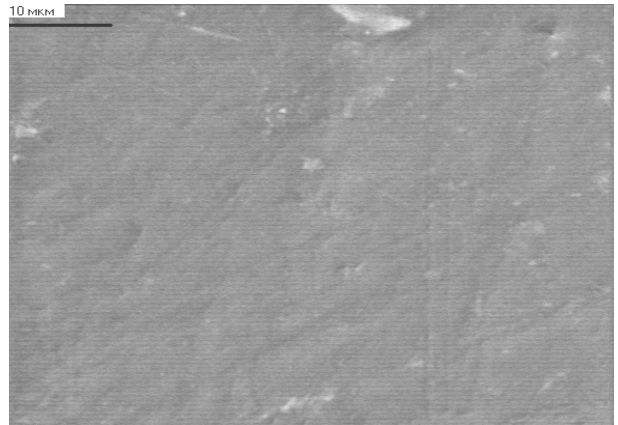
Рис. 1. Електроннограма поверхні акрилової пластмаси «Фторакс», контрольна група (а) РЕМ. Зб. X 2400
