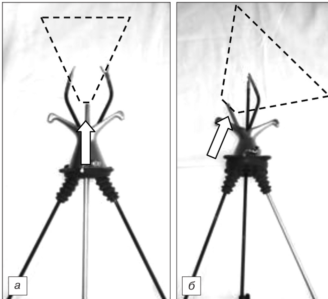
Рис. 3. Лапароскоп в положении прямого обзора (а) и бокового обзора и оптимальное расположение инструментов.
