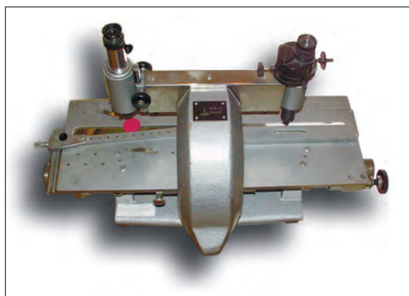
Рис. 2. Микроскоп-компаратор горизонтальный ИЗА-2 (Россия).
